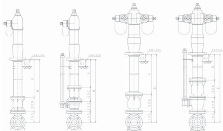
SC形 RSC形 SBC形 RSBC形 WPSOC形 WPRSOC形 WPSOBC形 WPRSOCBC形
