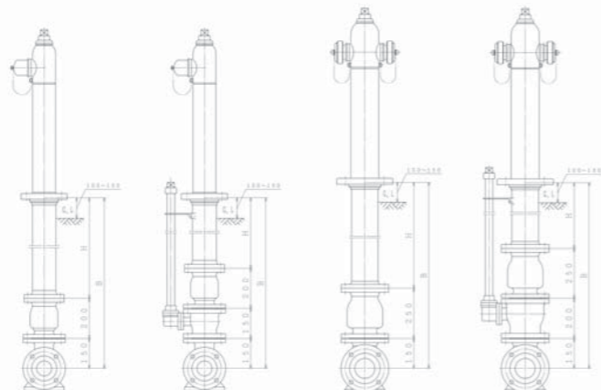
SC-2形 RSC-3形 SBC-2形 RSBC-3形 RSCW-6形 RSBCW-6形
