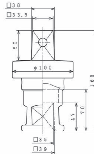
トルクリミッター本体
