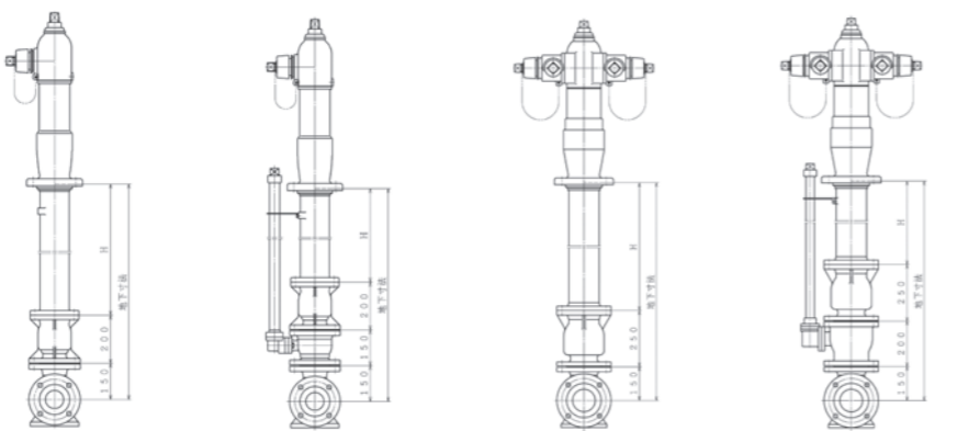
打倒式/単口 回転式/打倒式/単口 打倒式/双口 回転式/打倒式/双口 打倒式/副弁付/双口 回転式/打倒式/副弁付/双口
