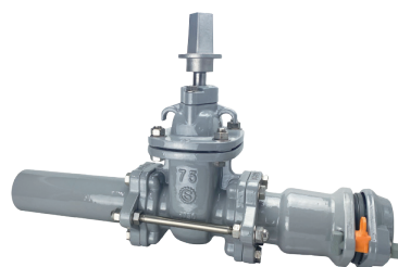
挿し口×塩ビ管受口 75mm
