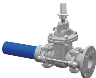
PE 管挿し口×フランジ 50 ~ 75mm
