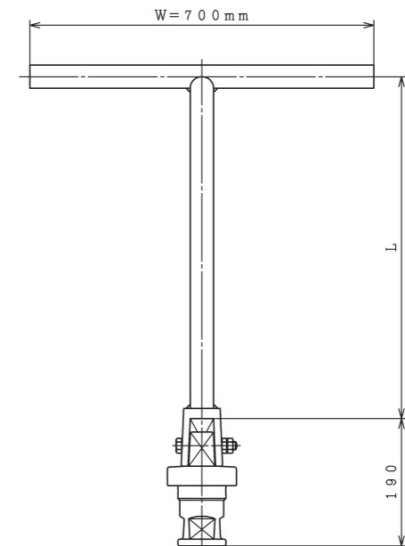
Tハンドル接続図
