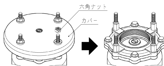
呼び径 150（スパナの呼び 24 mm）
