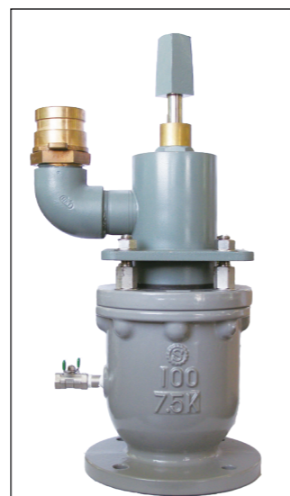
玉押器接続例
