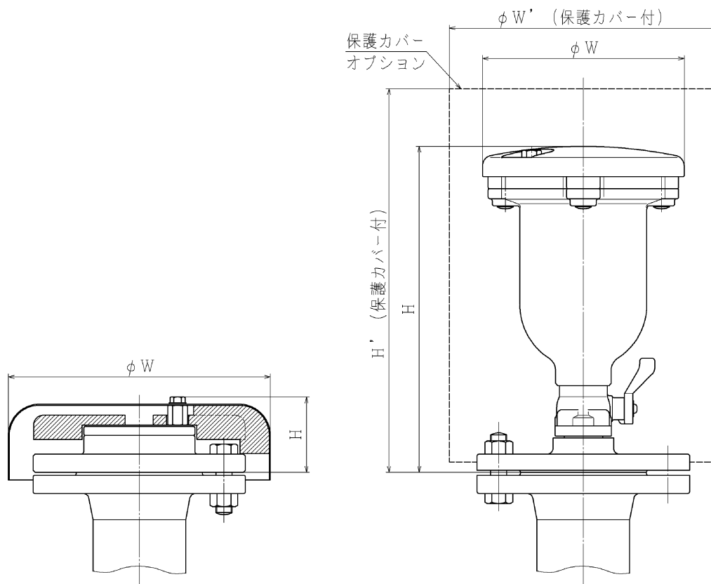
エアエルフ空気弁 呼び径 25
