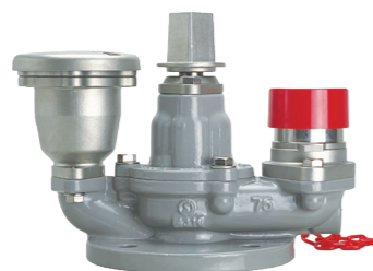
急速空気弁付 (ボールコック無)
