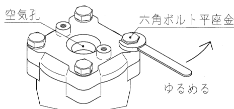
呼び径 25 以下 (スパナの呼び 17 mm)
