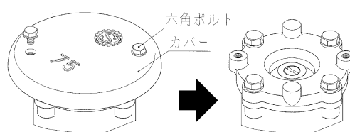
呼び径 75 (スパナの呼び 19 mm)
