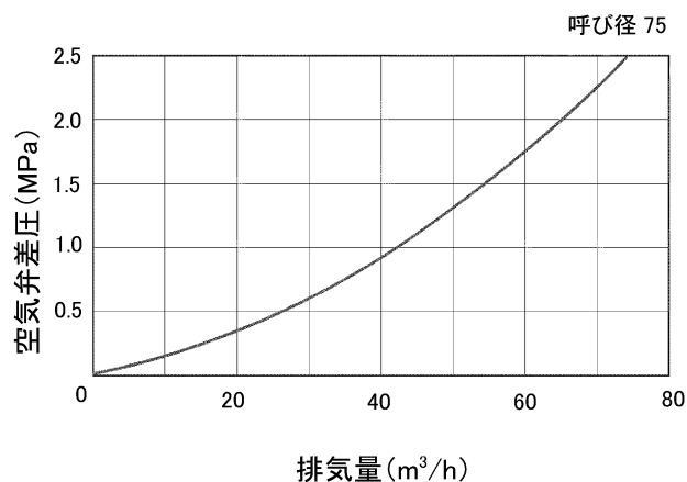
【圧力下排気特性】呼び径 75
