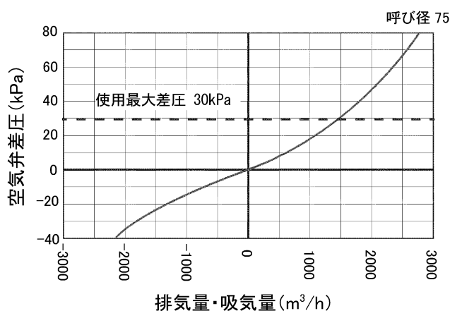
【多量排気・多量吸気特性】呼び径 75
