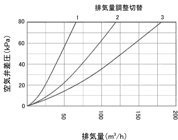
【ウォーターハンマー防止タイプ (NS) の排気・吸気特性】呼び径 75
