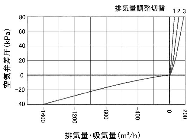
【ウォーターハンマー防止タイプ (NS) の排気・吸気特性】呼び径 75
